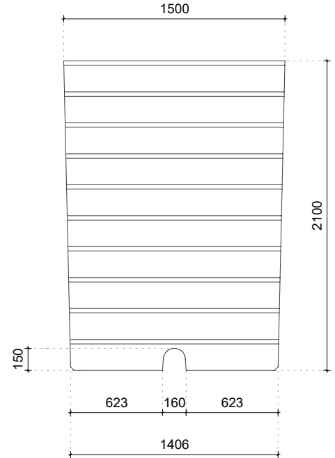
Vorderansicht
