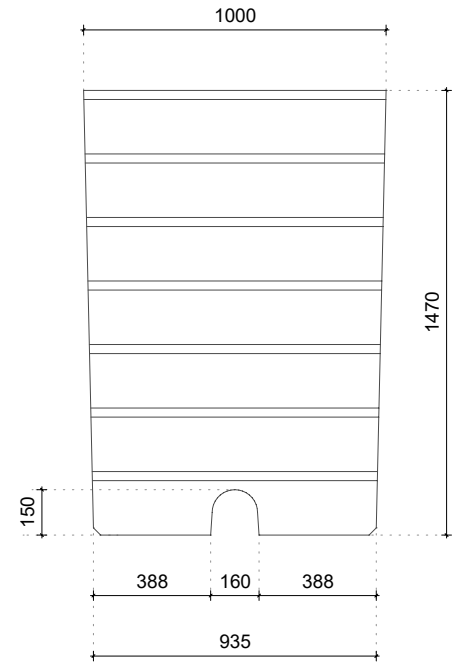
Vorderansicht
