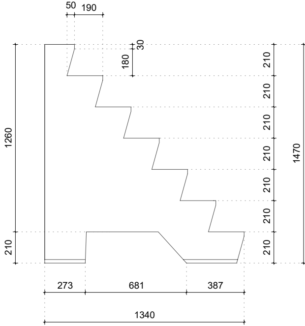
Seitenansicht
