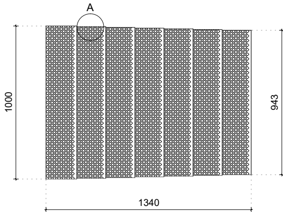
Draufsicht
